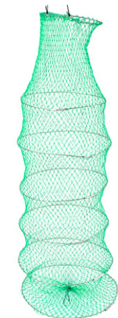
круглый (восьмерка), усиленный трос 1 x 19, 7 колец, 18 нитей
